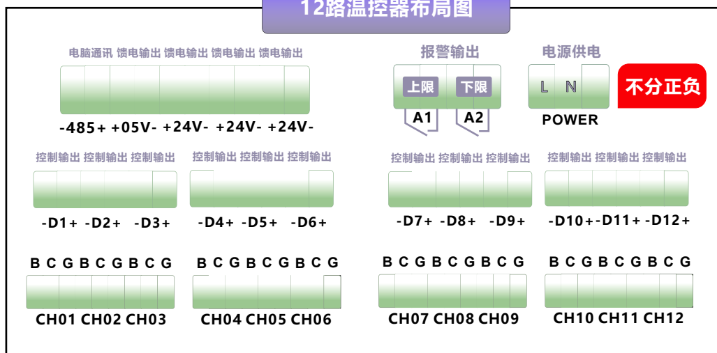
12路温控器布局图
