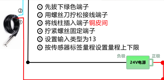
两线制液位变送器接线
