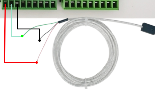
湿度传感器接线
