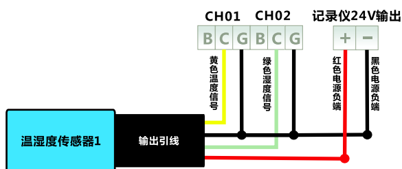
温湿度接线图
