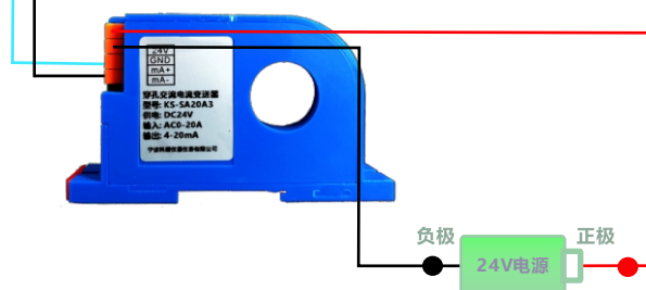
适用于四线制供电型变送器
