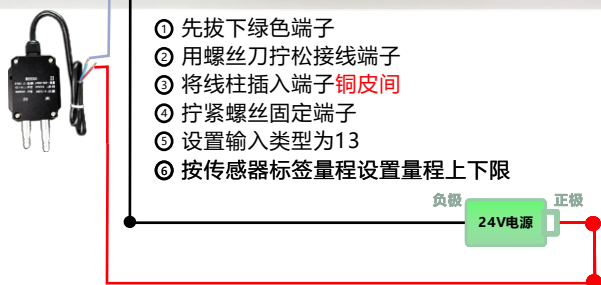
适用于两线制供电型变送器
