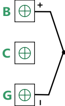
4-20mA接线 多个变压器接线时变压器正端并接在电源24V上 适用于两线制接线方式
