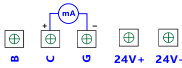
4-20mA接线 多个变压器接线时变压器正端并接在电源24V上 适用于两线制接线方式
