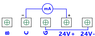
4-20mA接线
