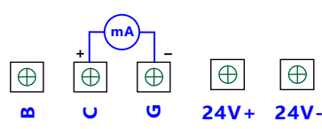
4-20mA接线
