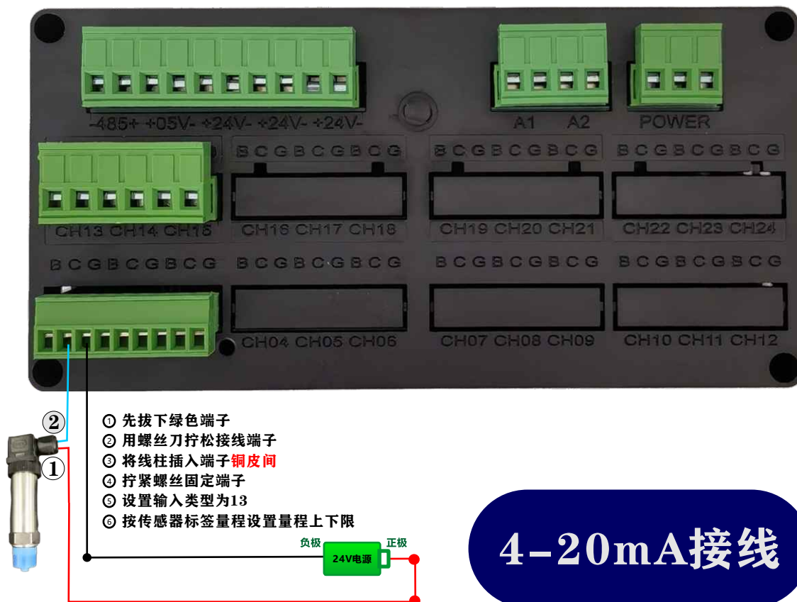
两线制压力变送器接线
